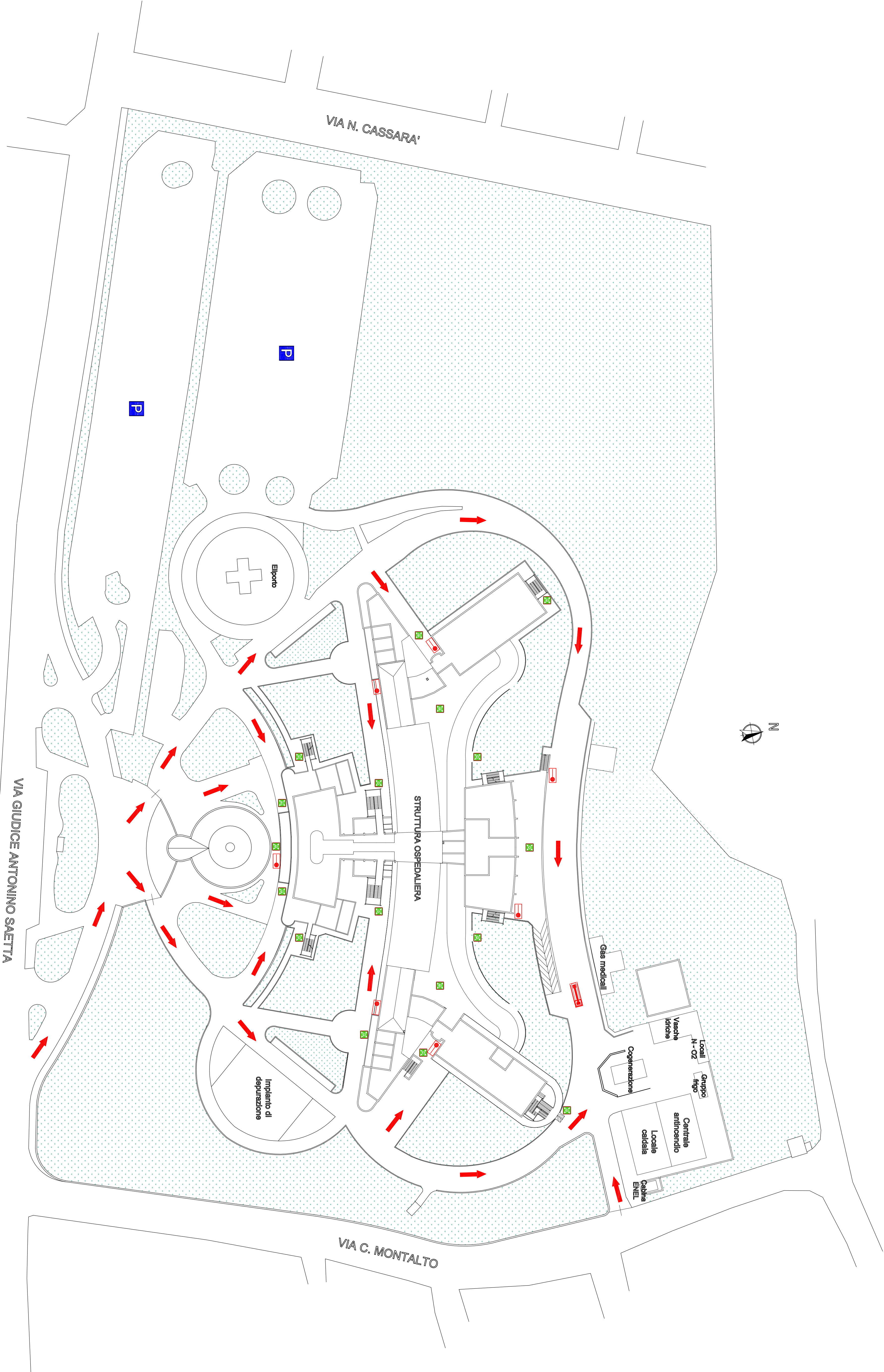
Planimetria generale Scala 1/500
